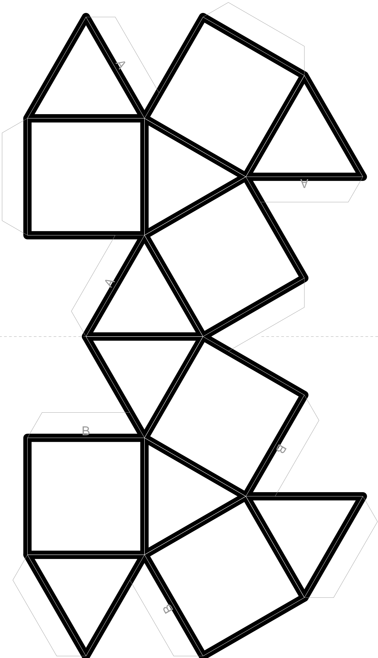
Pseudo-Kuboktaeder (3,3,4,4)*
